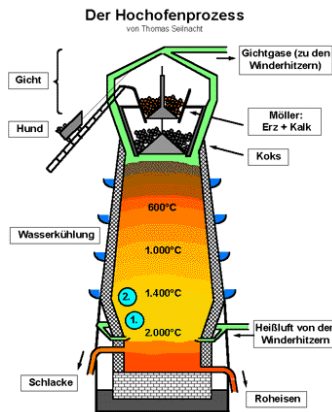
Abb. 5: Der Hochofenprozess
